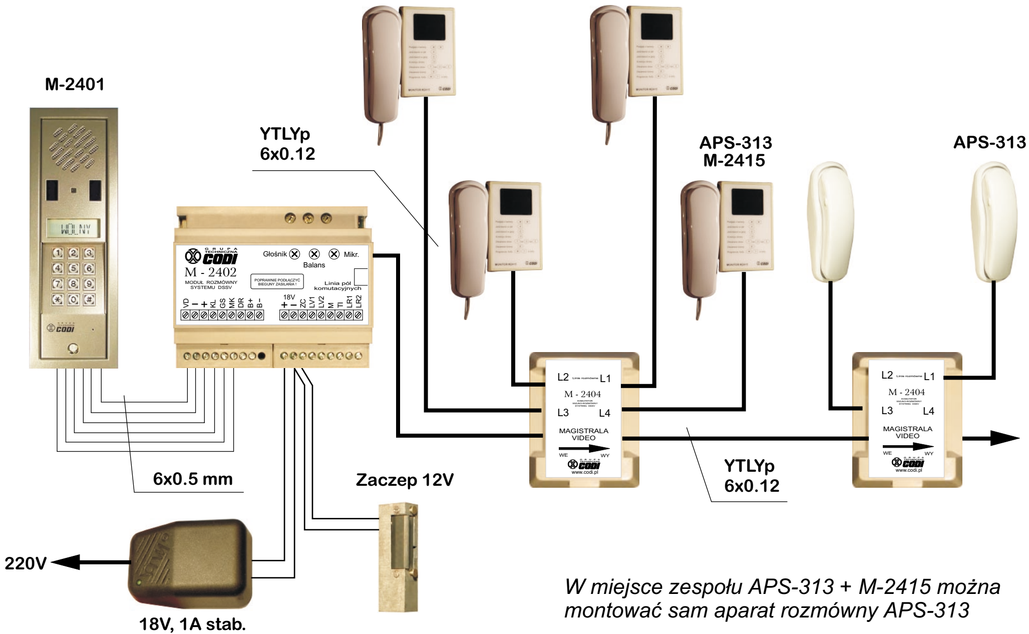
Schemat połączeń systemu DSSV dla pojedynczego obiektu z jednym wejściem
